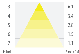
Suprema SQ 450
