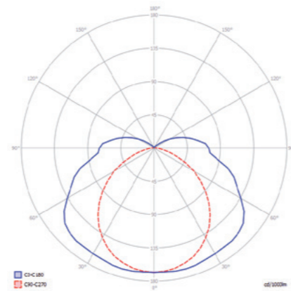
Herma 2x18
